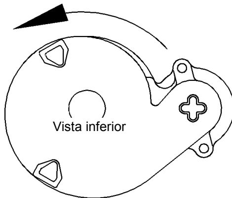
Fig. 1 – Rotación correcta del rotor, modelos trifásicos
